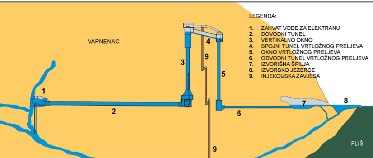
HPP Ombla, Dubrovnik
