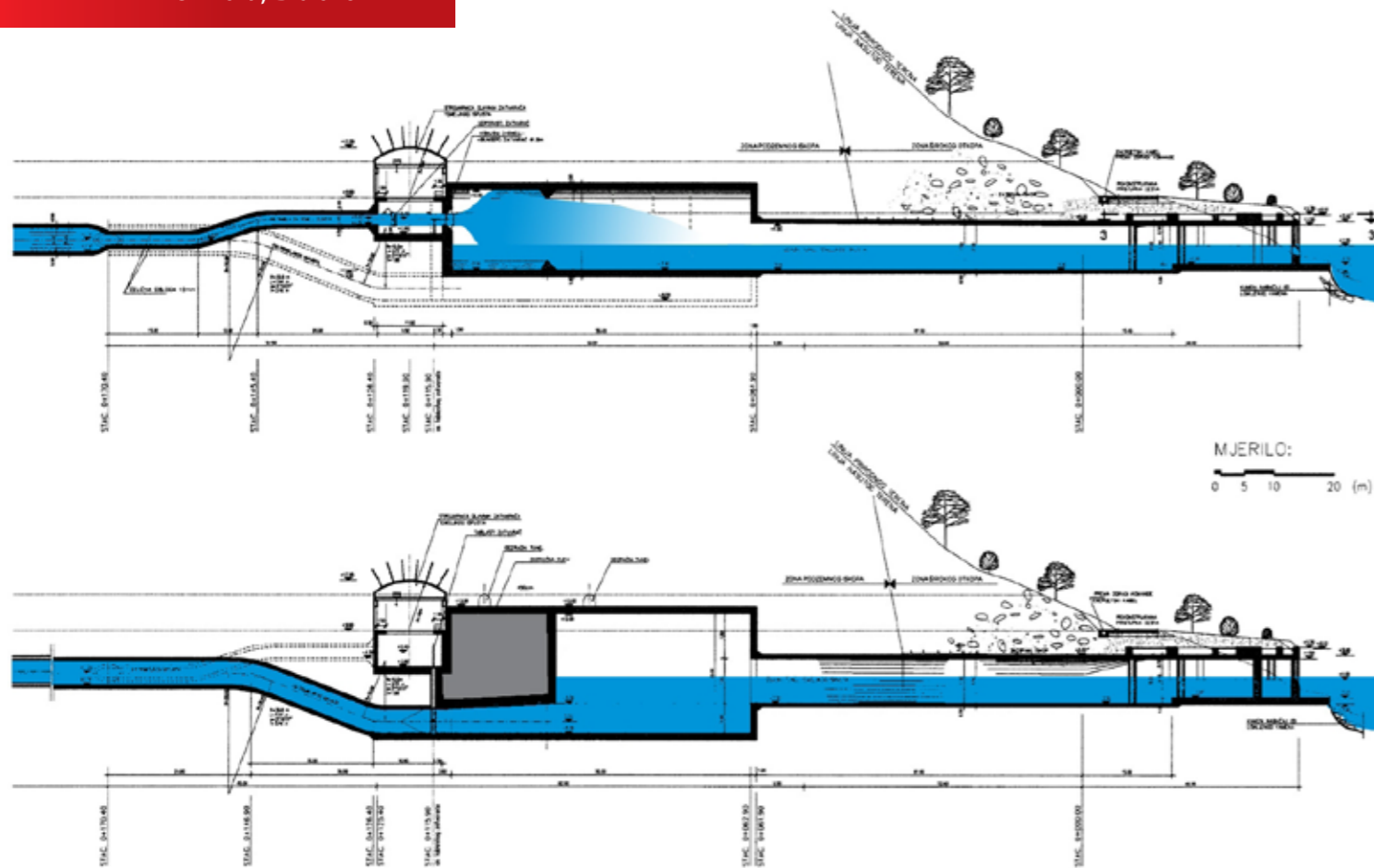
HPP Ombla, Dubrovnik
